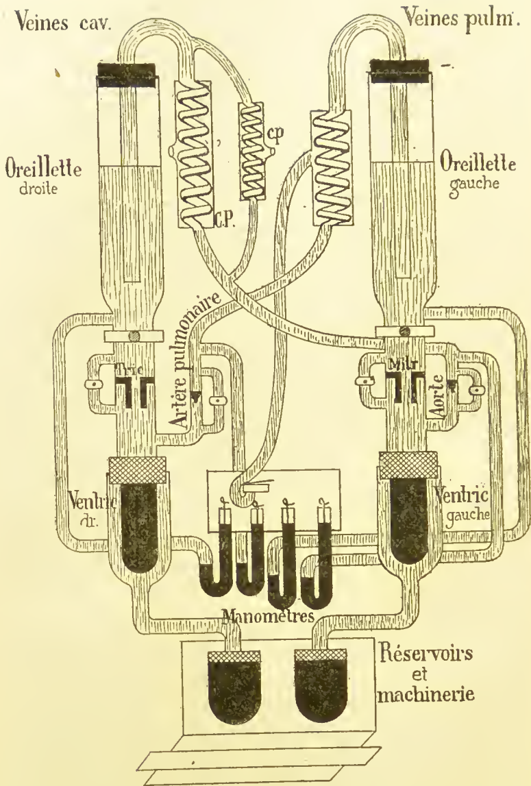
Fig. 25. — Schéma de la circulation pour l'étude des pressions de M. le Professeur von Basch.
